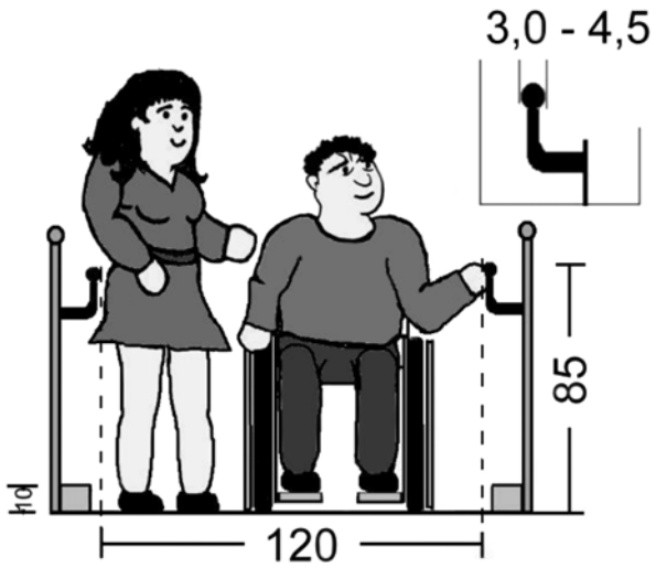
Rampe, Querschnitt
