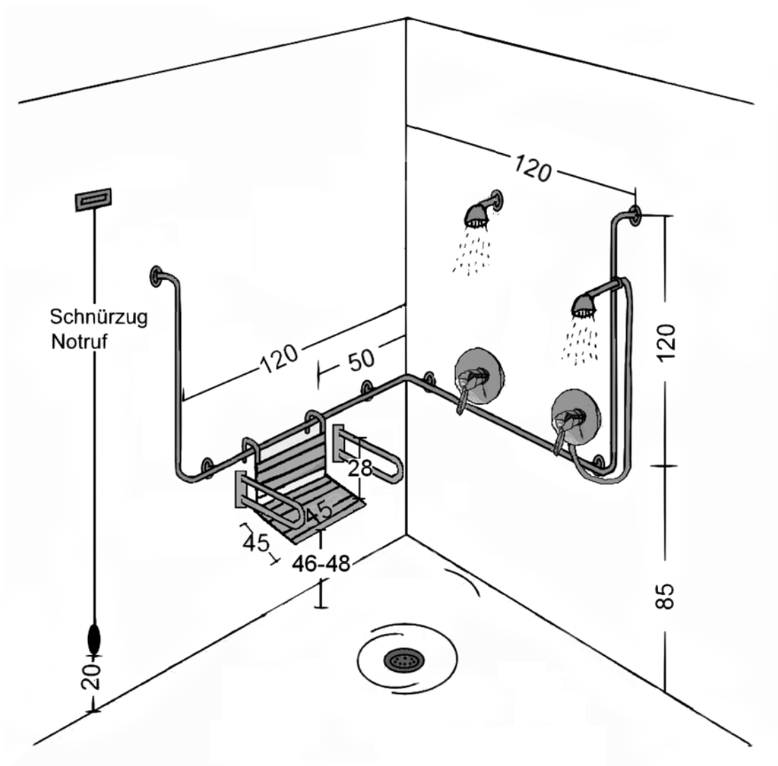
Anforderungen an eine barrierefreie Dusche
