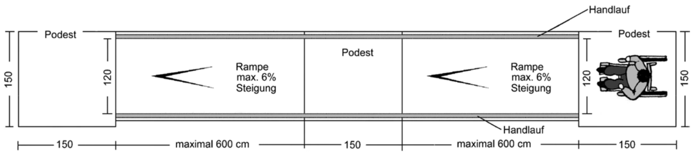
Rampe, Grundriss
