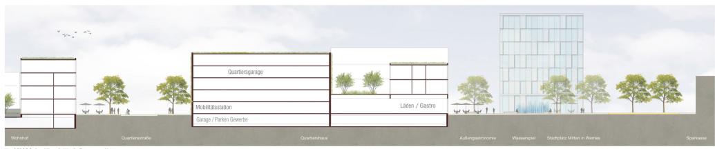
Nord-Süd Schnitt „Mitten in Werries“ M 1:200
